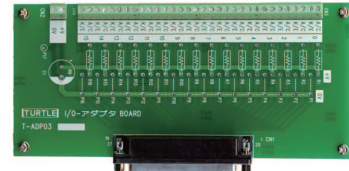
アダプタボードT-ADP03Z(オプション)
