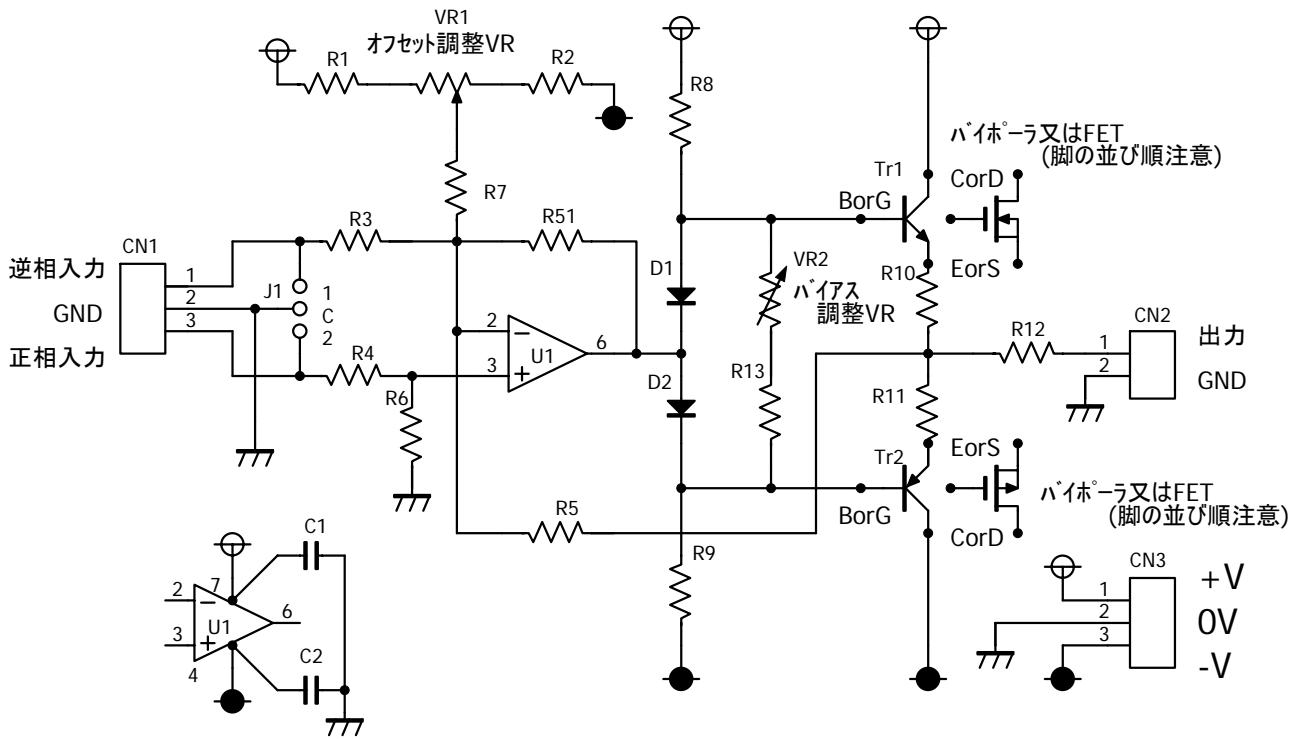
T-AMP03回路図
